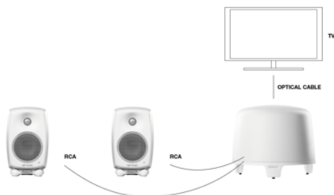
例 1：テレビのデジタル出力からの接続
